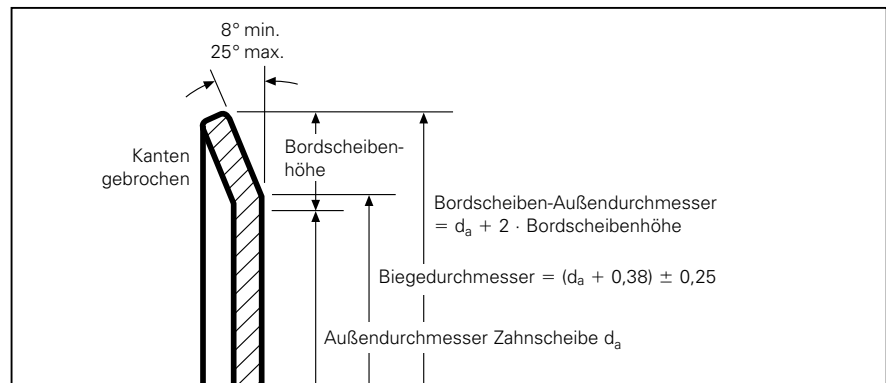
Bordscheibe
