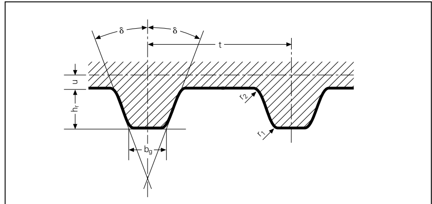
Abwälzfräser für Evolventen-Zähne
