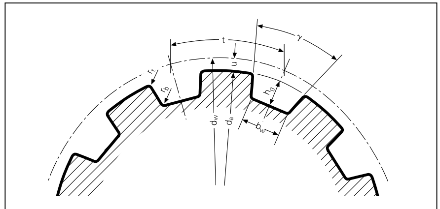
Zahnlücke mit geraden Flanken
