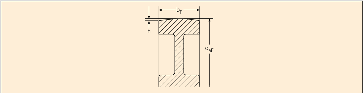
Abb./Fig. 8 Wölbhöhe an einer Flachscheibe / Curvature on a flat pulley
